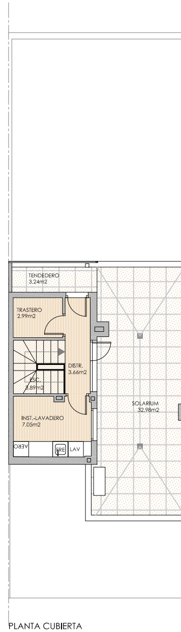
PLANTA CUBIERTA
