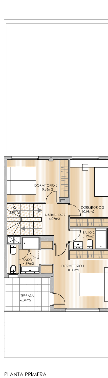
PLANTA PRIMERA
